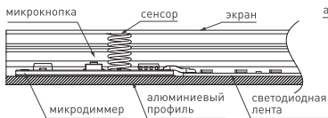
Рисунок 2. Микродиммер, установленный в профиль. Вид сбоку.
