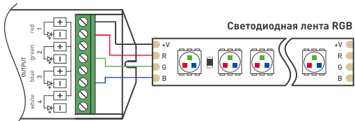
Рисунок 2. Подключение ленты RGB (3сН).
