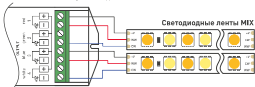
Рисунок 3. Подключение ленты MIX (2сН).
